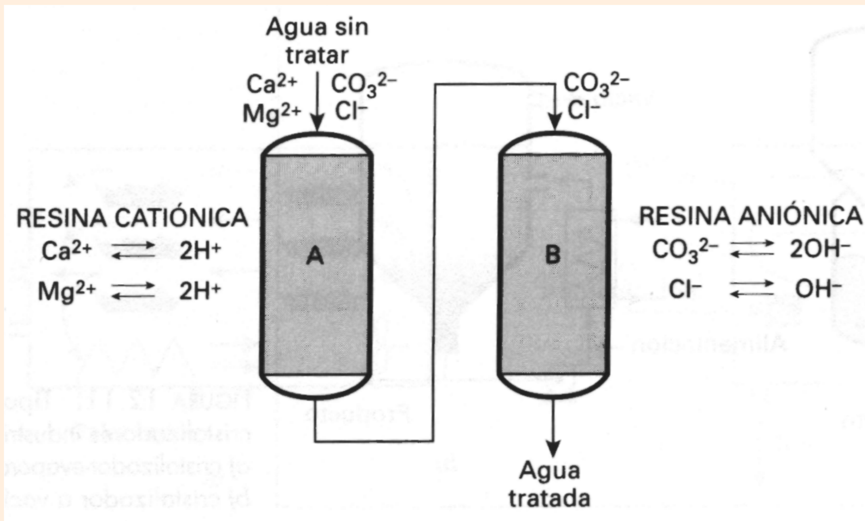
Figura 5.10: Intercambio iónico.
