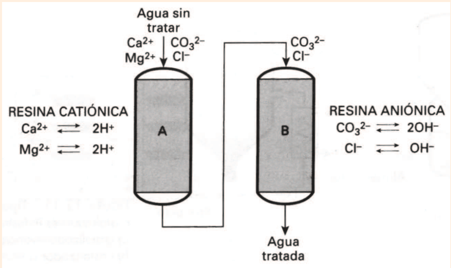
Figura 5.10: Intercambio iónico.
